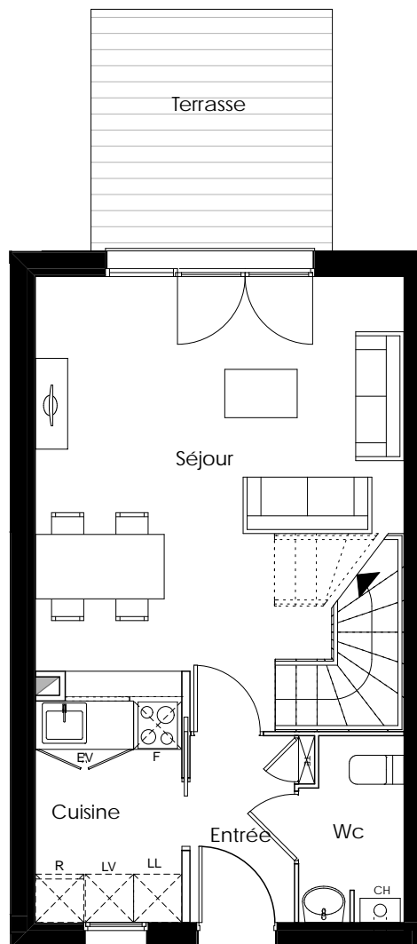
PLAN RDC
